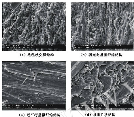
图 2 青海软玉的扫描电镜图
