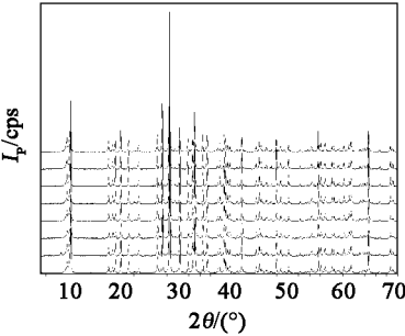
图 1 软玉 X 射线衍射图谱
