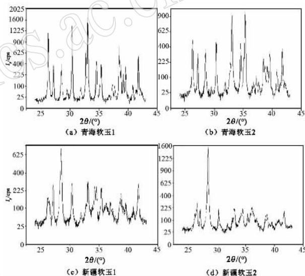
图 3 青海软玉与和田玉结晶度 X 射线衍射分析图谱
