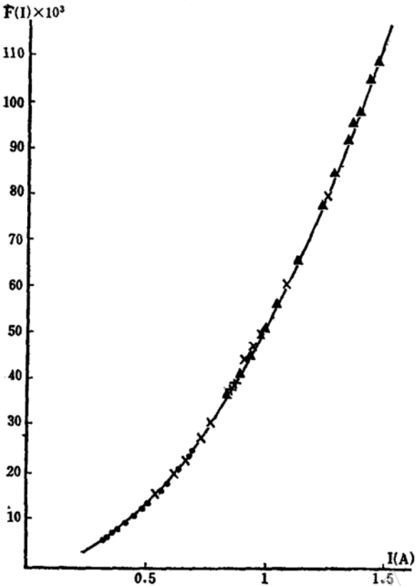
图 2 I—F 工作曲线
