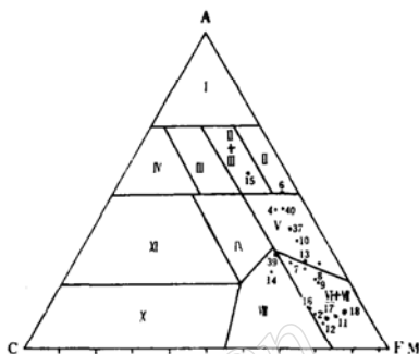
图1 A-C-FM图解
