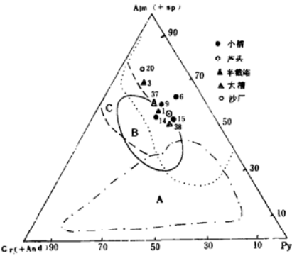
图 5 石榴石在铁铝榴石(Alm) + 锰铝榴石(sp) - 钙铝榴石(Gr) + 钙铁榴石(And) - 镁铝榴石Py三角图上的投影 麻粒岩(点线区) 榴辉岩(A、B、C区) *
