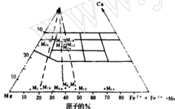
图4 辉石的化学成分在Ca—Mg—Fe( \text{Fe}^{2+} + \text{Fe}^{3+} + \text{Mn} )三角图中的投影 (1)
