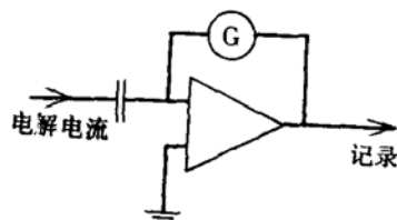
图5 半微分路原理图 (G表示梯型网络)
